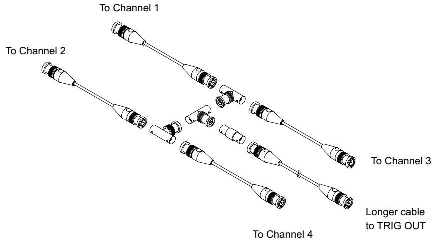
그림 52 4 채널 오실로스코프용 사용자 교정 케이블
