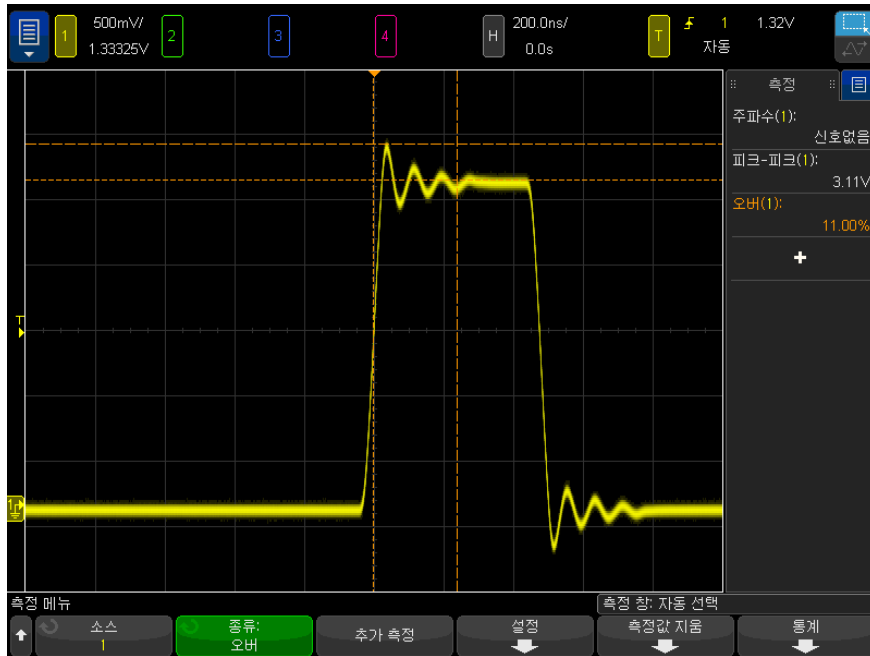
그림 49 자동 오버슈트 측정
