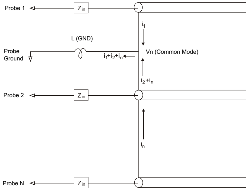
그림 26 공통 모드 입력 전압 모델
