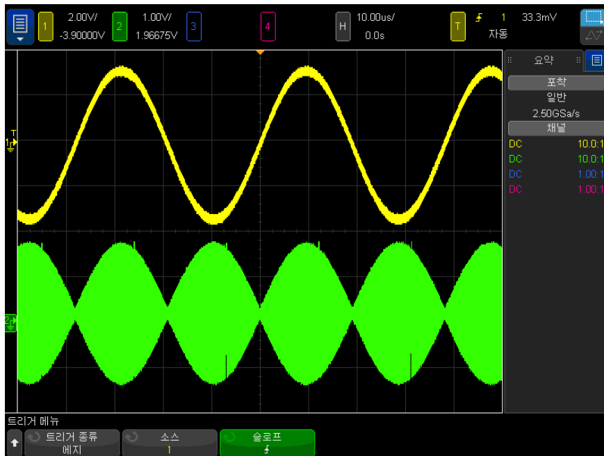
그림 27 100% 명암으로 표시된 진폭 변조
