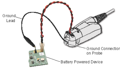
그림 47 N2820A 프로브를 사용하여 배터리로 전원이 공급되는 장치에서 측정
