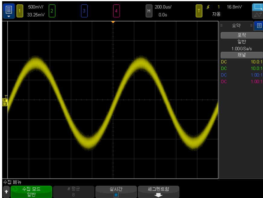
그림 40 표시되는 파형의 무작위 노이즈
