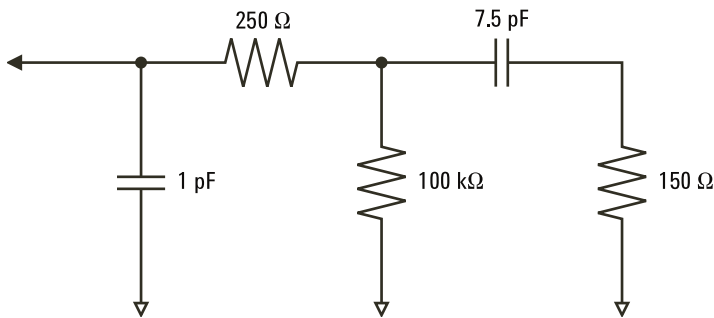
그림 24 고주파 프로브 등가 회로
