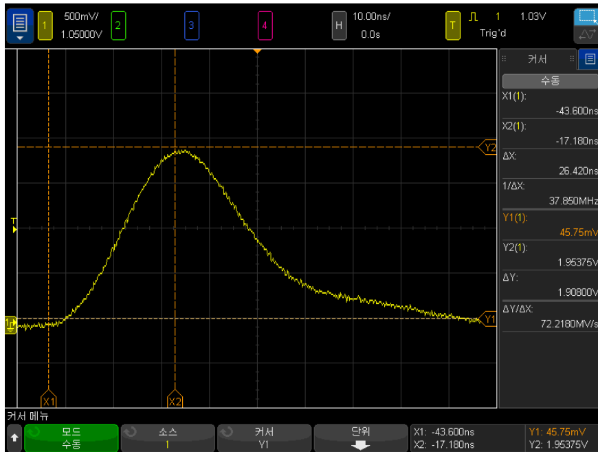
그림 42 중간 임계값 포인트 이외의 펄스 폭을 측정하는 데 사용되는 커서
