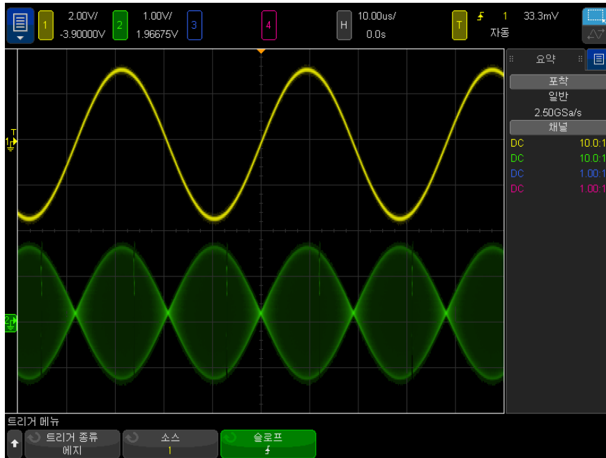
그림 28 40% 명암으로 표시된 진폭 변조
