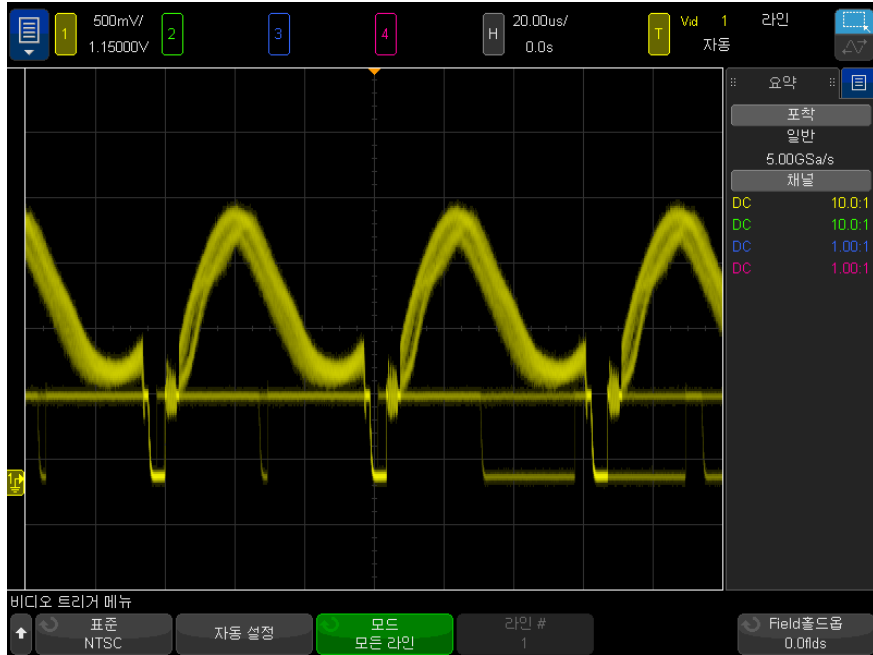
그림 30 모든 라인에 트리거링
