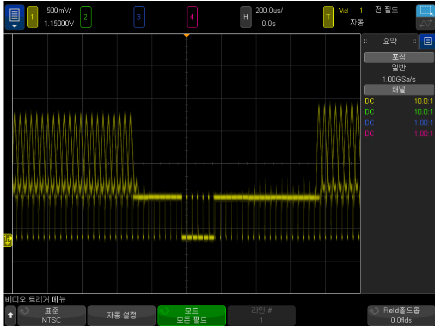
그림 32 모든 필드에 트리거링
