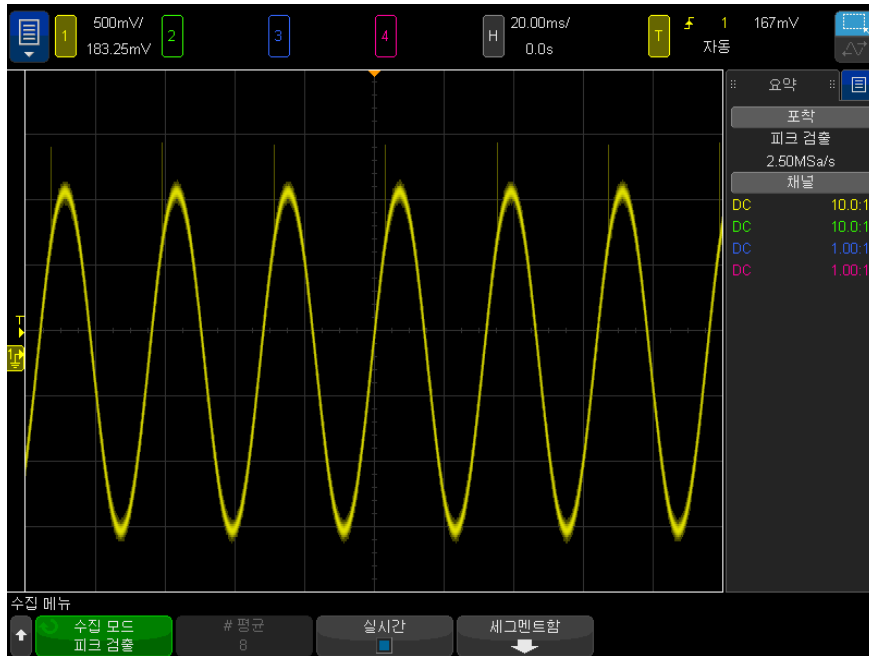
그림 39 글리치가 포함된 사인파 , 피크 검출 모드
