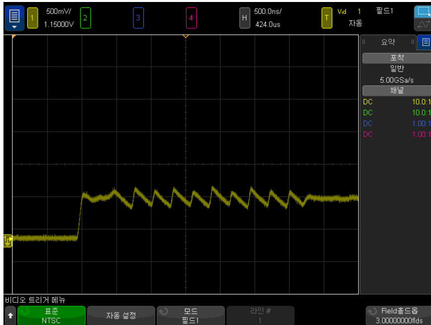
그림 34 필드 홀드오프를 사용하여 컬러 필드 1 또는 3에 동기화 (필드 1 모드)
