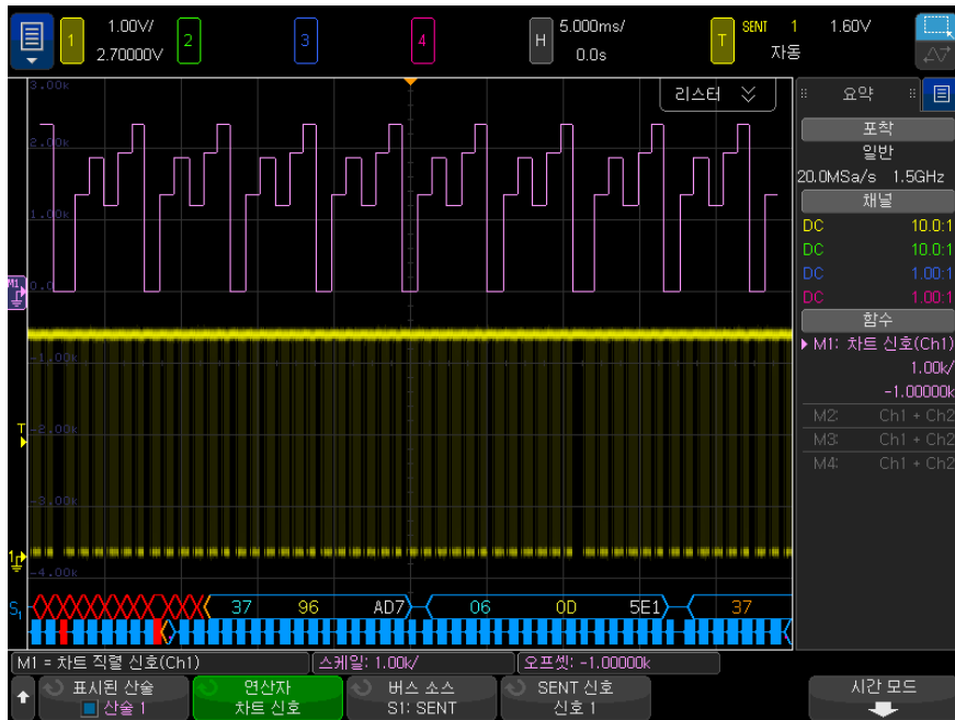
그림 21 차트 직렬 신호의 예
