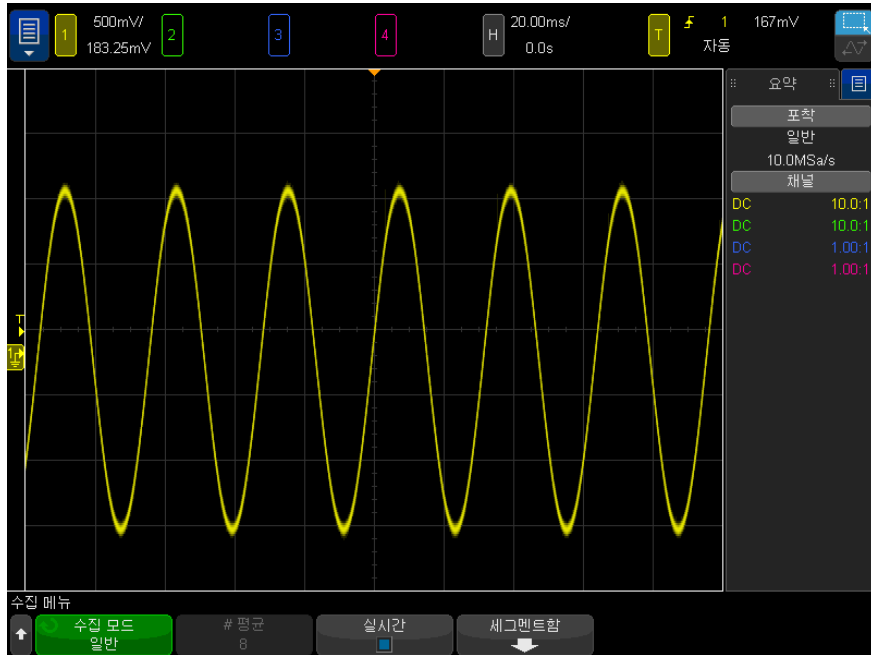
그림 38 글리치가 포함된 사인파, 일반 모드
