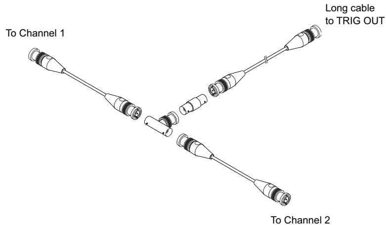
그림 51 2 채널 오실로스코프용 사용자 교정 케이블
