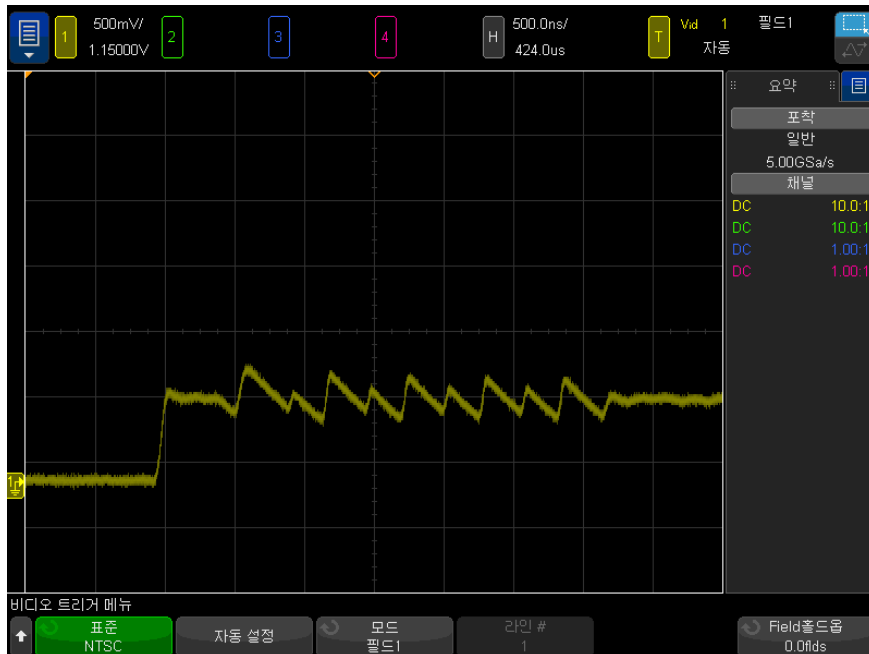
그림 33 컬러 필드 1과 컬러 필드 3에 교대로 트리거링
