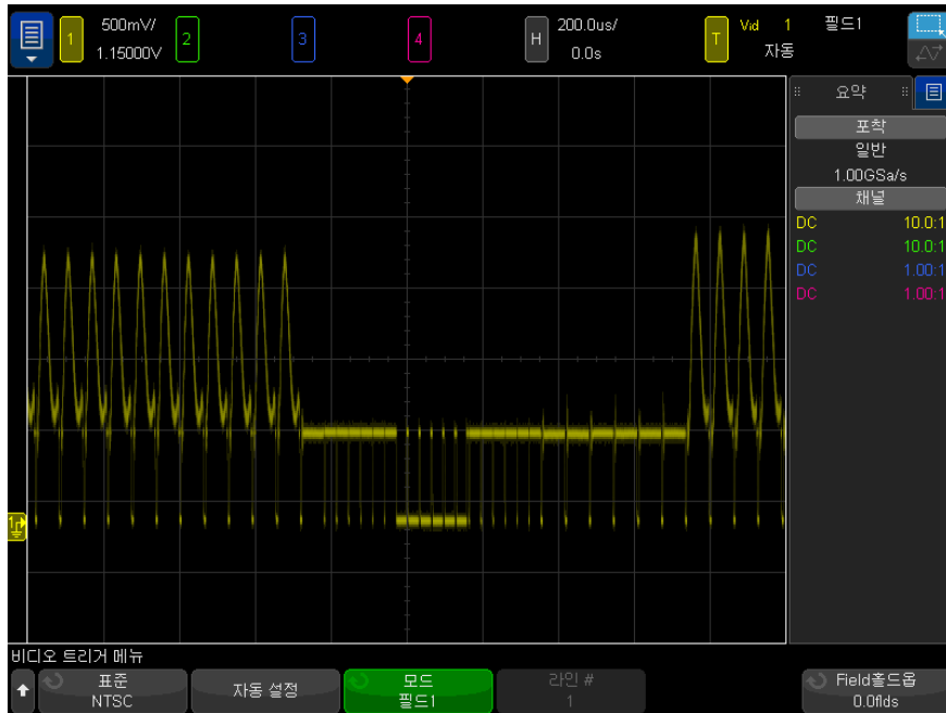
그림 31 필드 1 에 트리거링
