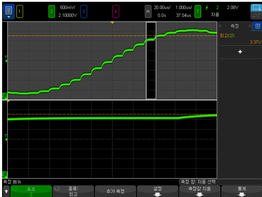
그림 48 최고값 측정을 위한 영역 격리
