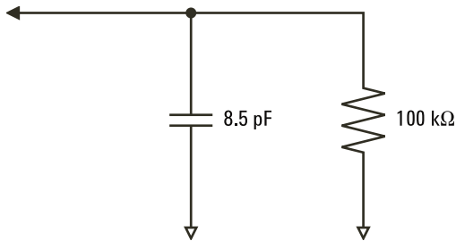
그림 23 DC 및 저주파 프로브 등가 회로
