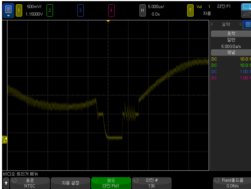
그림 29 예 : 라인 136 에 트리거링
