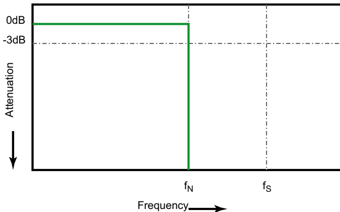
그림 36 이론적인 Brick-Wall 주파수 응답
