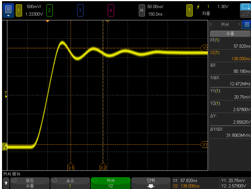
그림 43 펄스 링잉의 주파수를 측정하는 커서
