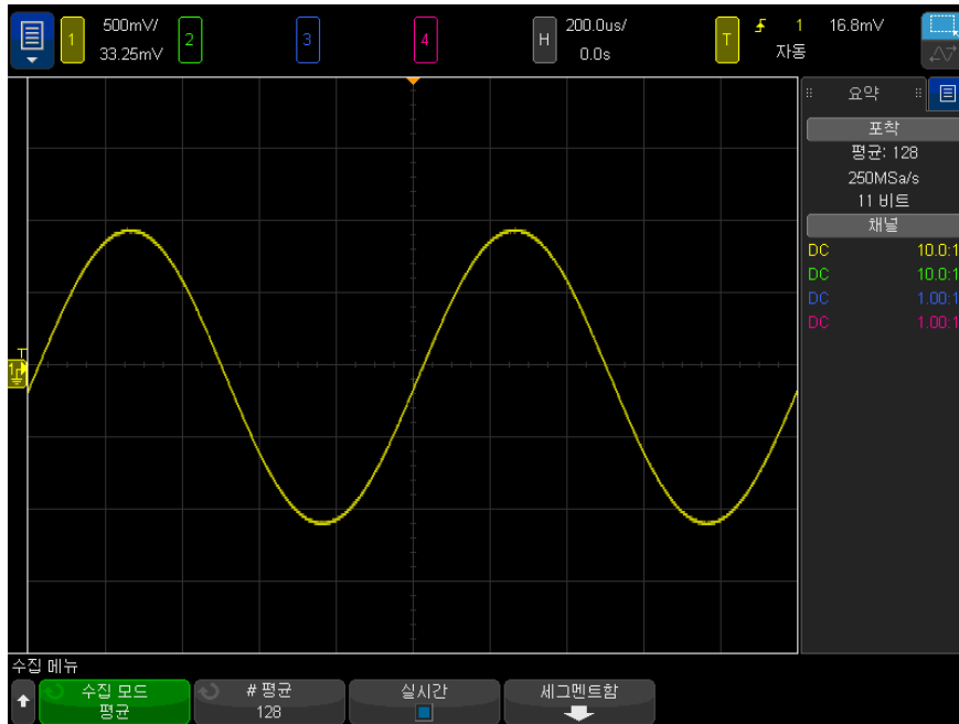
그림 41 무작위 노이즈를 줄이는 데 128 개의 평균이 사용됨
