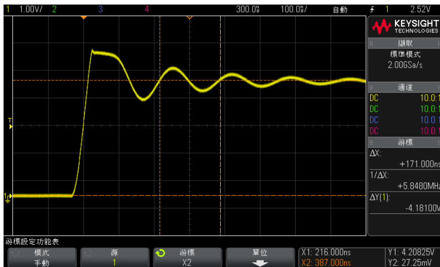
圖 41 量測脈波瞬變頻率的游標
