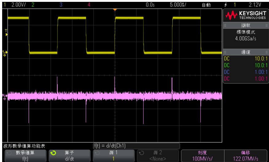
圖 7 微分函數的範例
