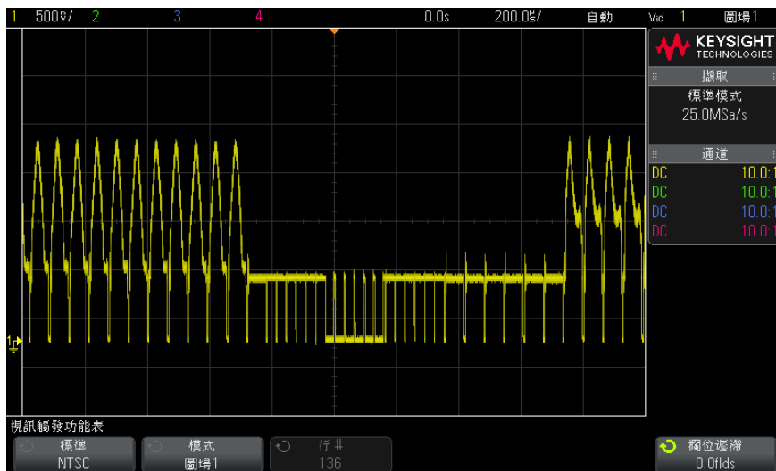
圖 29 針對圖場 1 進行觸發
