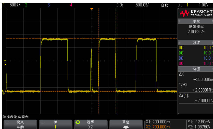
圖 43 使用游標量測脈波寬度
