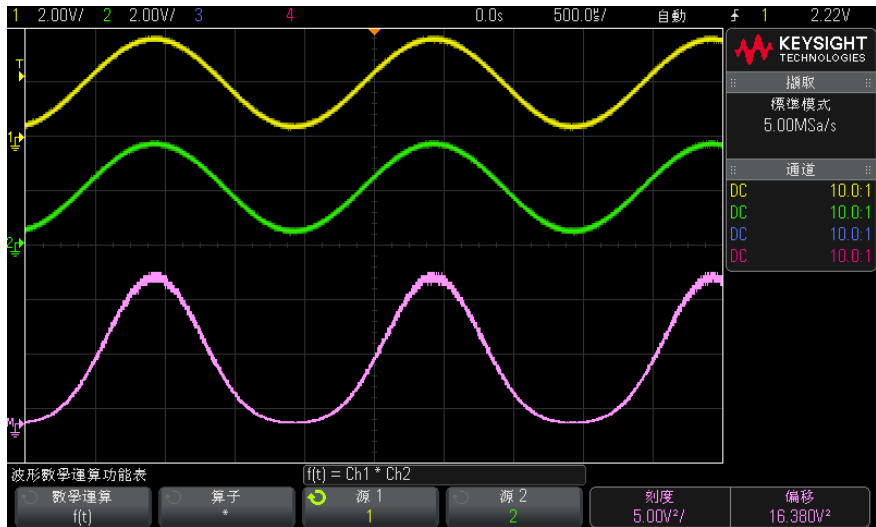
圖 6 通道 1 乘通道 2 範例
