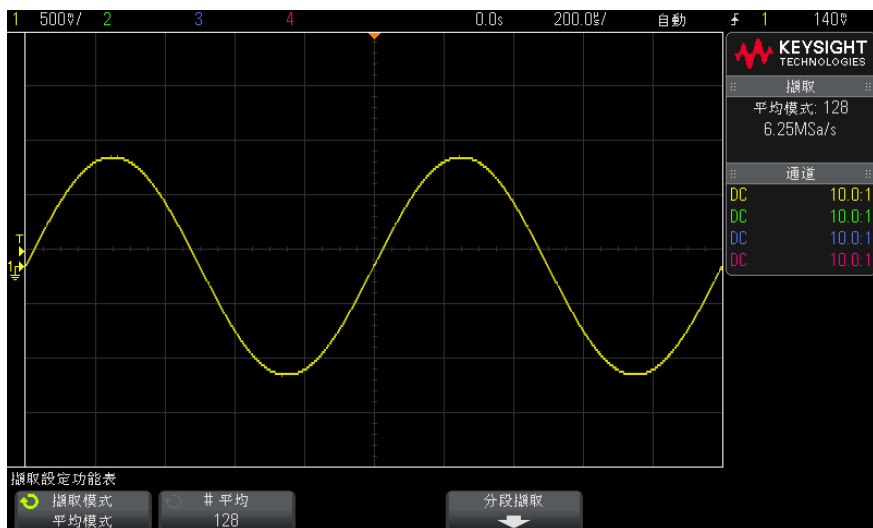
圖 39 對 128 個擷取進行平均以減少隨機雜訊
