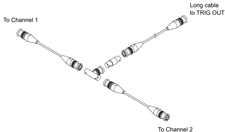
圖 49 2 通道示波器的使用者校準纜線
