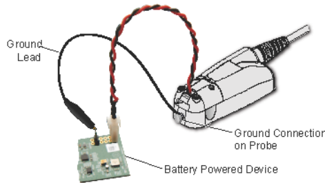
圖 45 使用 N2820A 測試棒對電池供電裝置進行量測
