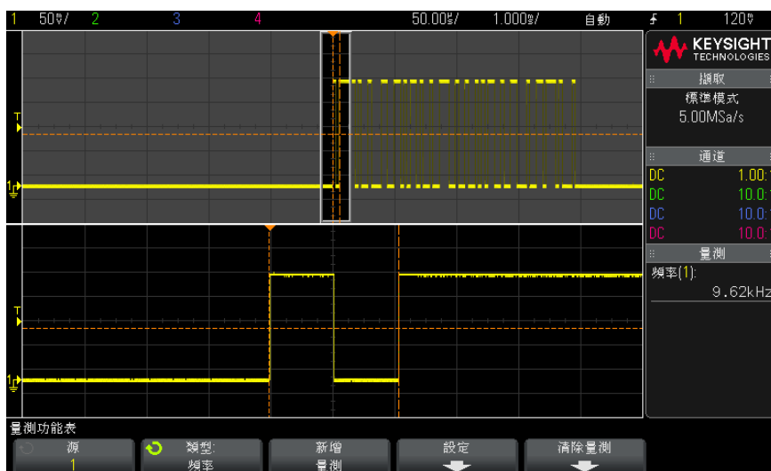
圖 48 區隔頻率量測的事件
