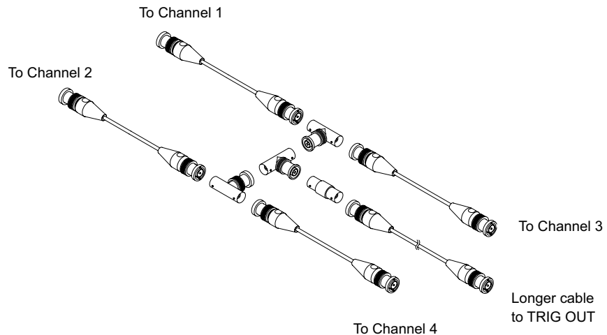
圖 50 4 通道示波器的使用者校準纜線
