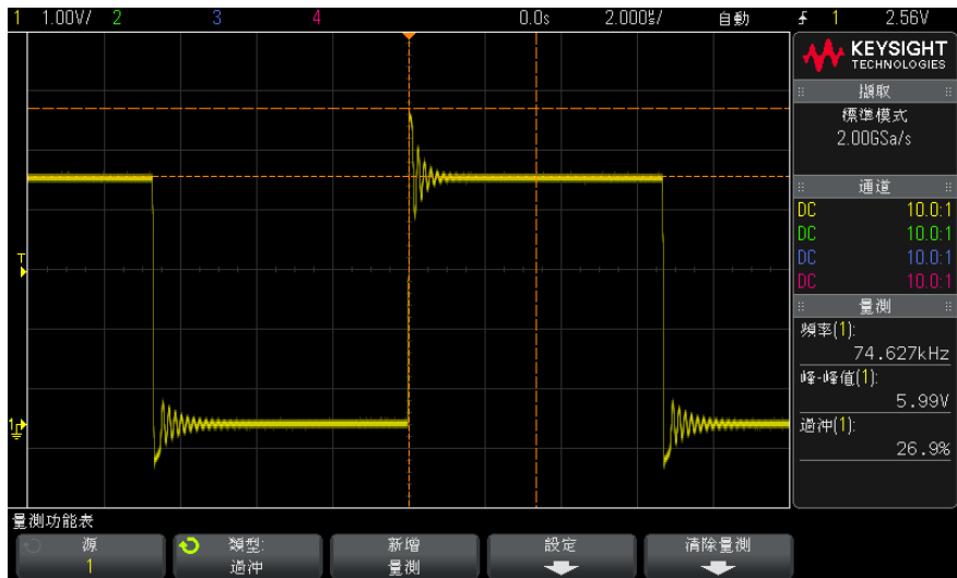
圖 47 自動過沖量測
