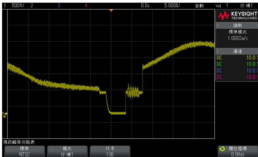
圖 27 範例：針對第 136 行進行觸發
