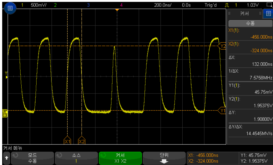
그림 46 커서를 함께 움직여 펄스 폭 변동 검사
