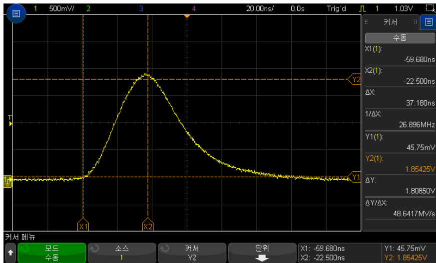
그림 42 중간 임계값 포인트 이외의 펄스 폭을 측정하는 데 사용되는 커서
