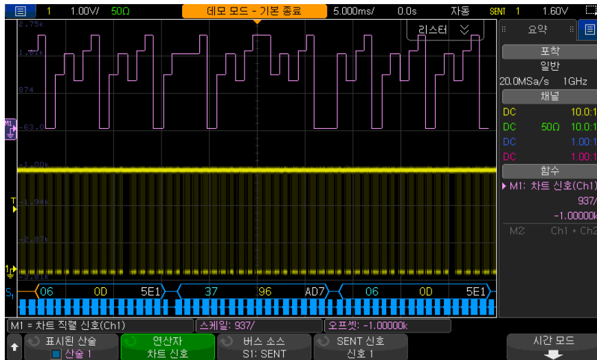
그림 21 차트 직렬 신호의 예
