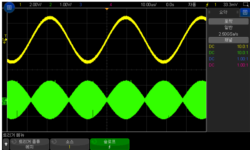
그림 27 100% 명암으로 표시된 진폭 변조
