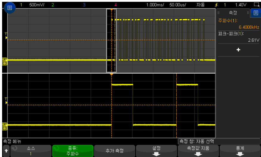
그림 50 주파수 측정을 위한 이벤트 거리
