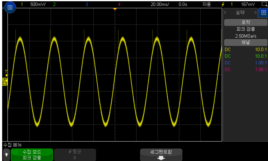
그림 39 글리치가 포함된 사인파, 피크 검출 모드
