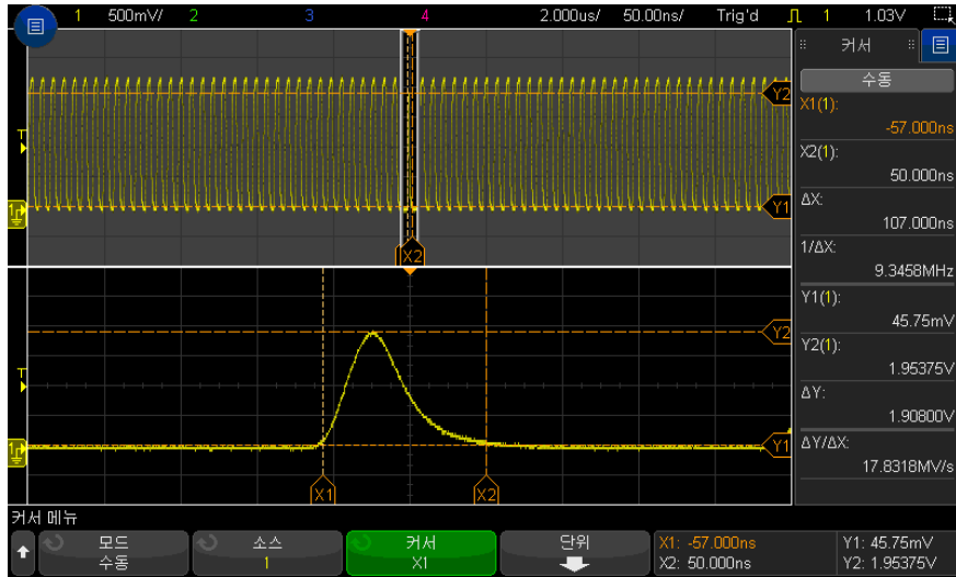
그림 44 줌 윈도우를 추적하는 커서
