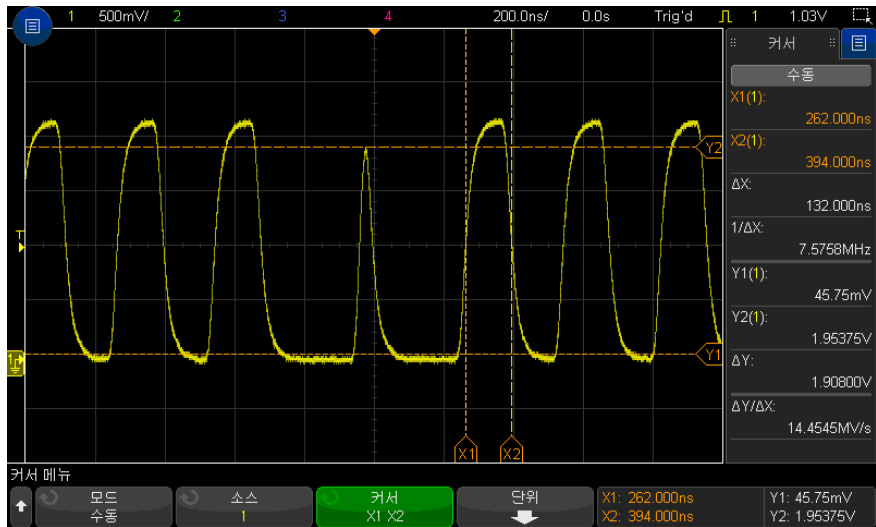
그림 45 커서를 사용한 펄스 폭 측정
