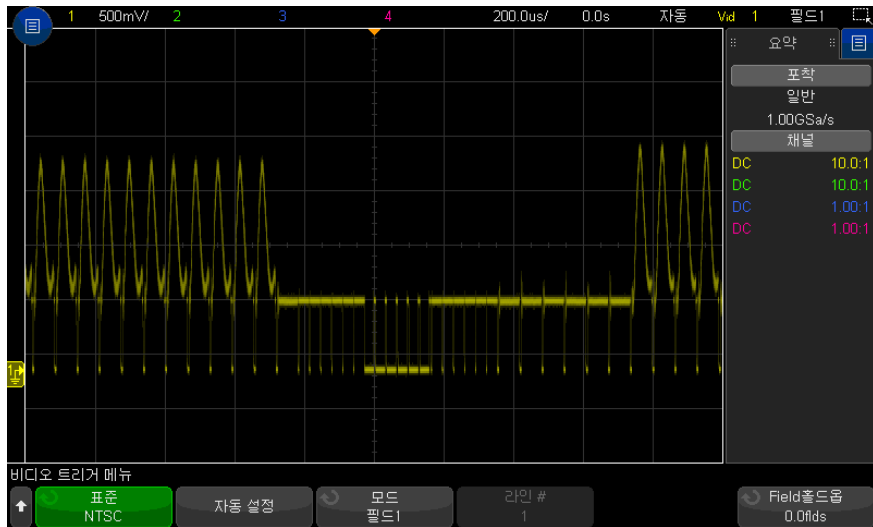
그림 31 필드 1 에 트리거링
