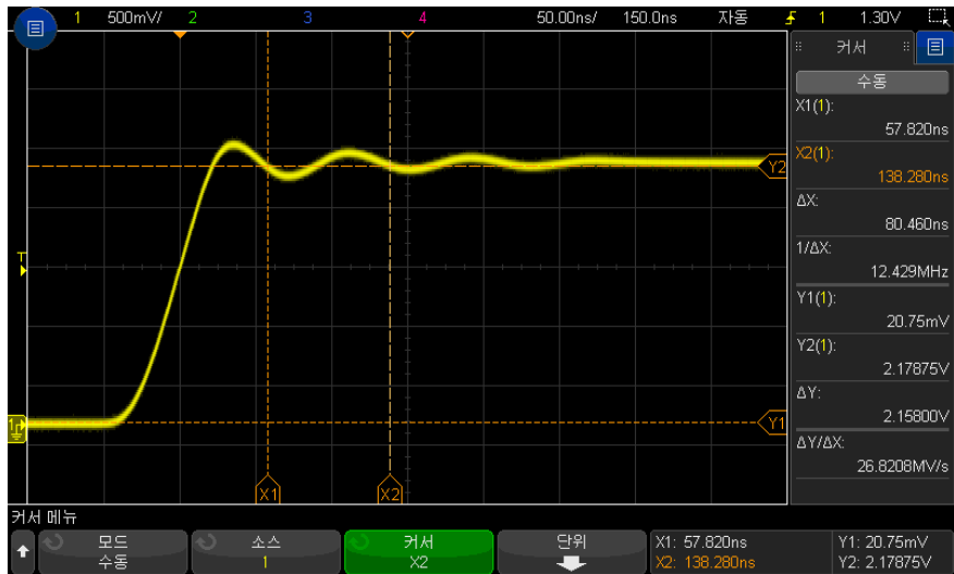
그림 43 펄스 링잉의 주파수를 측정하는 커서
