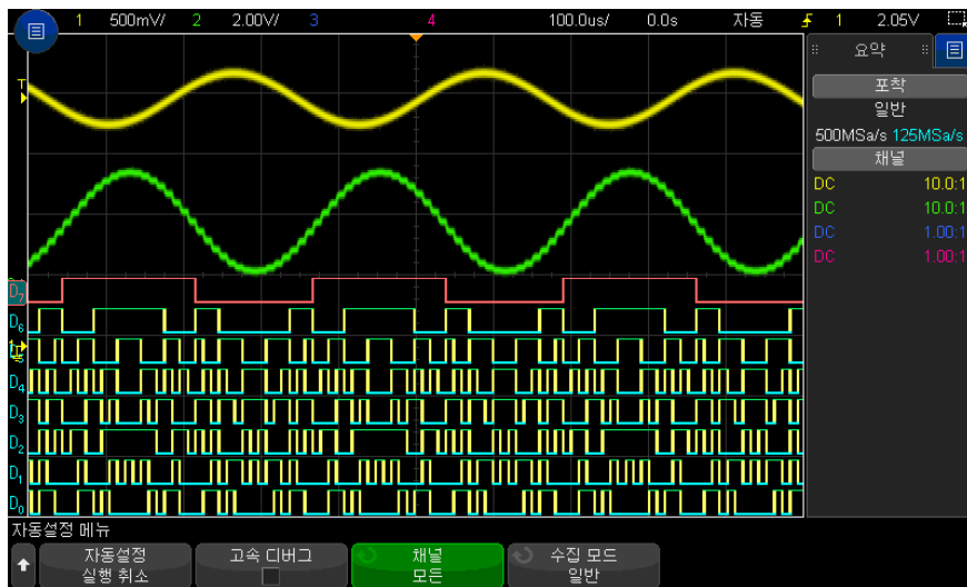
그림 22 예 : 디지털 채널의 자동 스케일 (MSO 모델에 한함)
