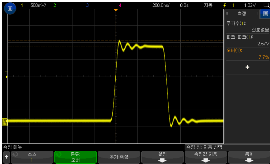
그림 49 자동 오버슈트 측정
