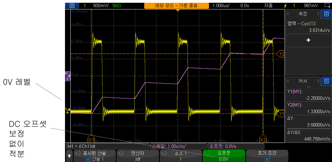
그림 9 신호 오프셋이 없는 적분
