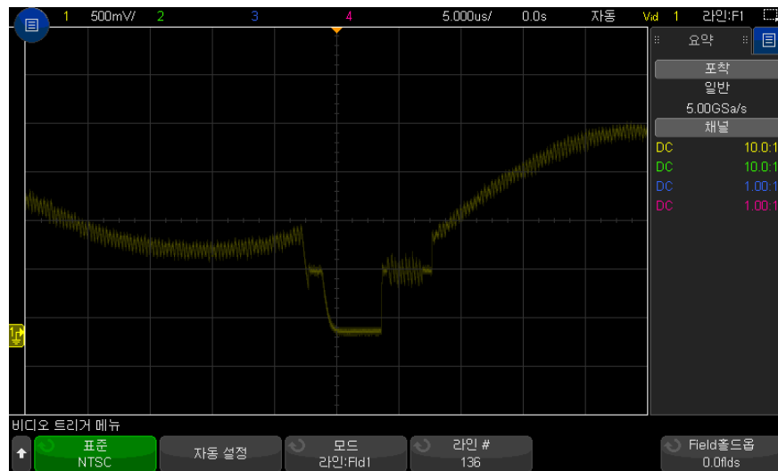
그림 29 예 : 라인 136 에 트리거링
