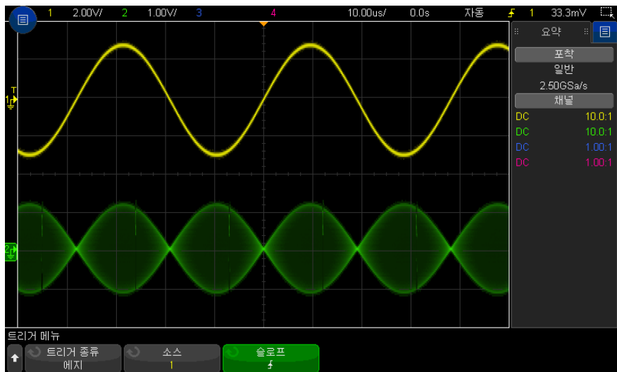
그림 28 40% 명암으로 표시된 진폭 변조
