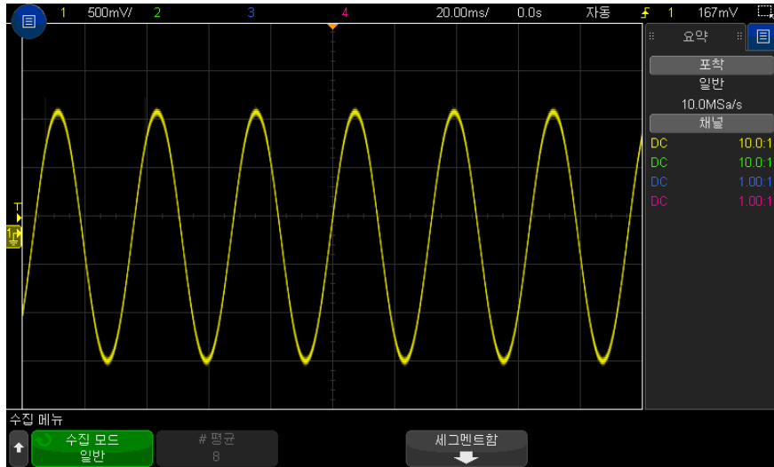
그림 38 글리치가 포함된 사인파, 일반 모드
