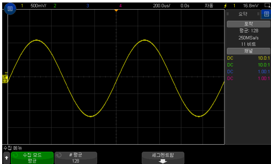
그림 41 무작위 노이즈를 줄이는 데 128 개의 평균이 사용됨
