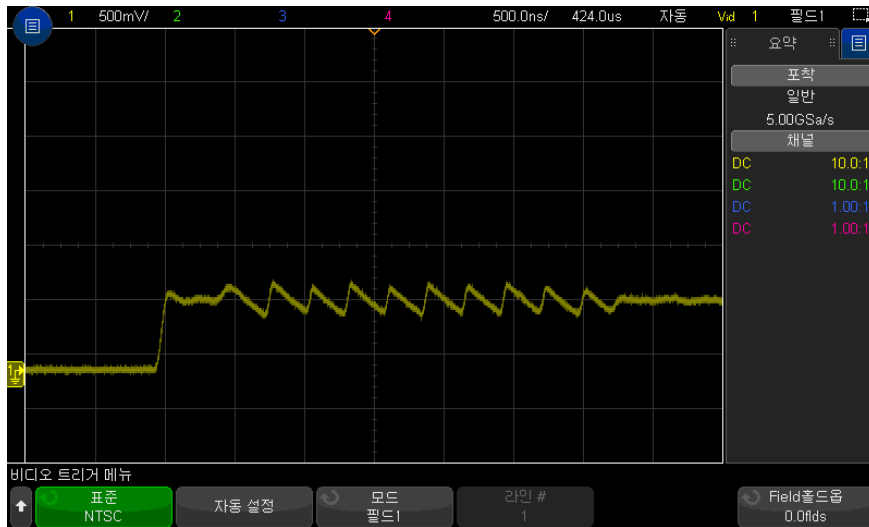
그림 33 컬러 필드 1 과 컬러 필드 3 에 교대로 트리거링
