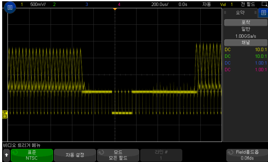
그림 32 모든 필드에 트리거링
