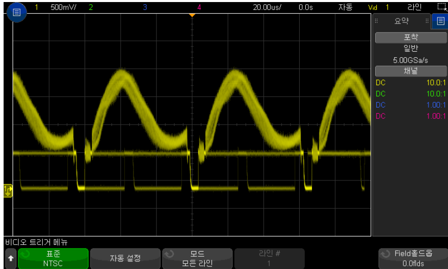
그림 30 모든 라인에 트리거링
