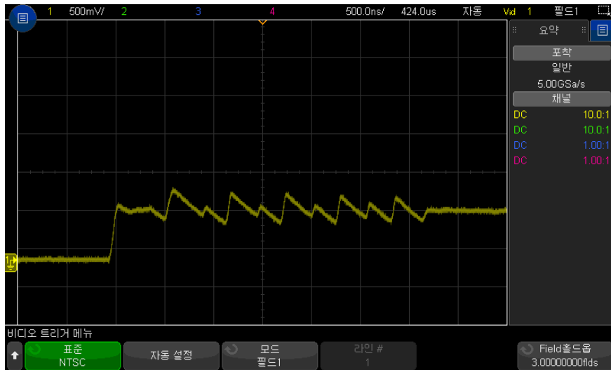
그림 34 필드 홀드오프를 사용하여 컬러 필드 1 또는 3에 동기화 (필드 1 모드)
