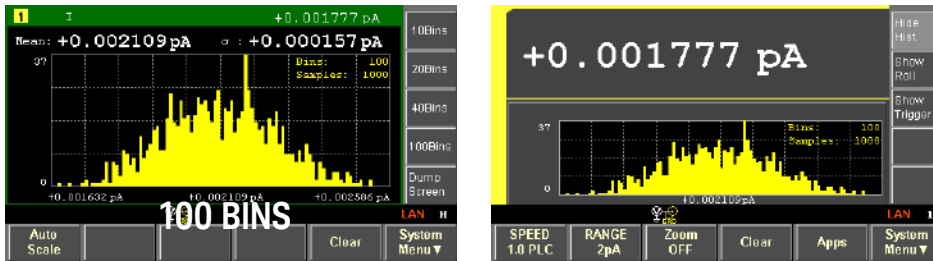
히스토그램 뷰
