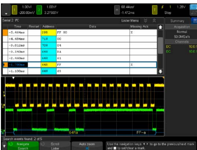
그림 11. 에러 조건 검색을 사용하여 4000 X-시리즈는 I²C 시리얼 버스 내에서 확인 응답이 없는 5개 지점을 신속하게 찾아냈습니다. 이 탐색 기능은 에러와 줌을 반복적으로 검색하여 에러 패킷을 보여줍니다.
