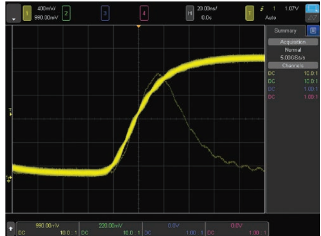
그림 3. 4000 X-시리즈는 100만 파형 주기마다 단 한번 발생하는 글리치를 수집합니다.
