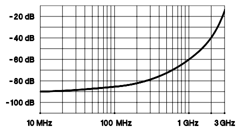
クロストーク (75Ω)
