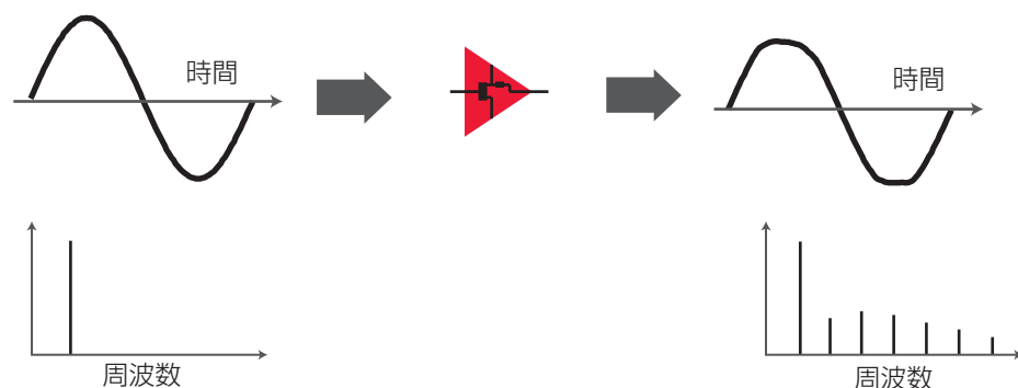
図4. ノンリニア歪み
