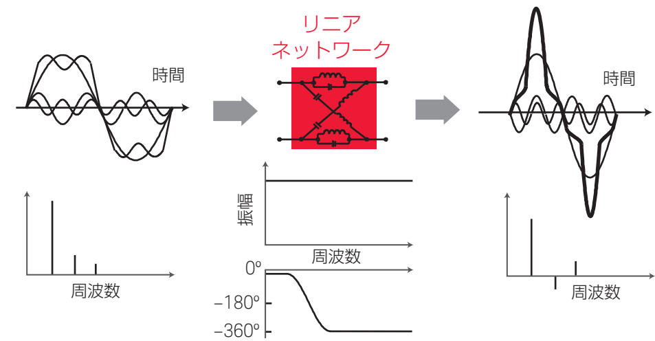
図3. 周波数による位相の変動
