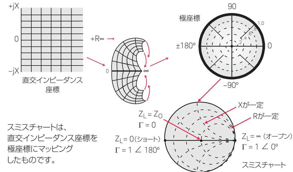
図6. スミスチャート
