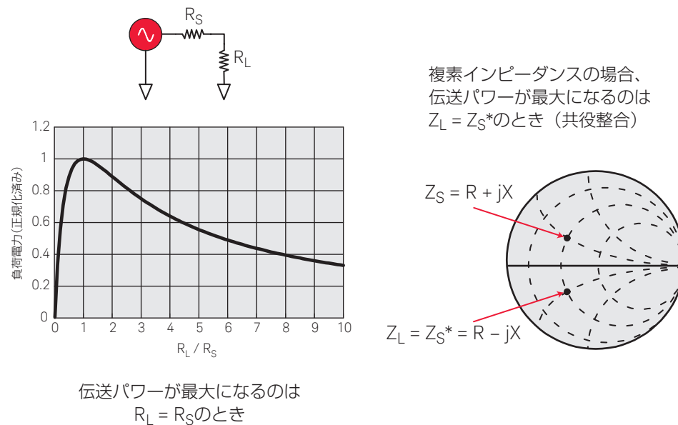
図7. パワー伝送
