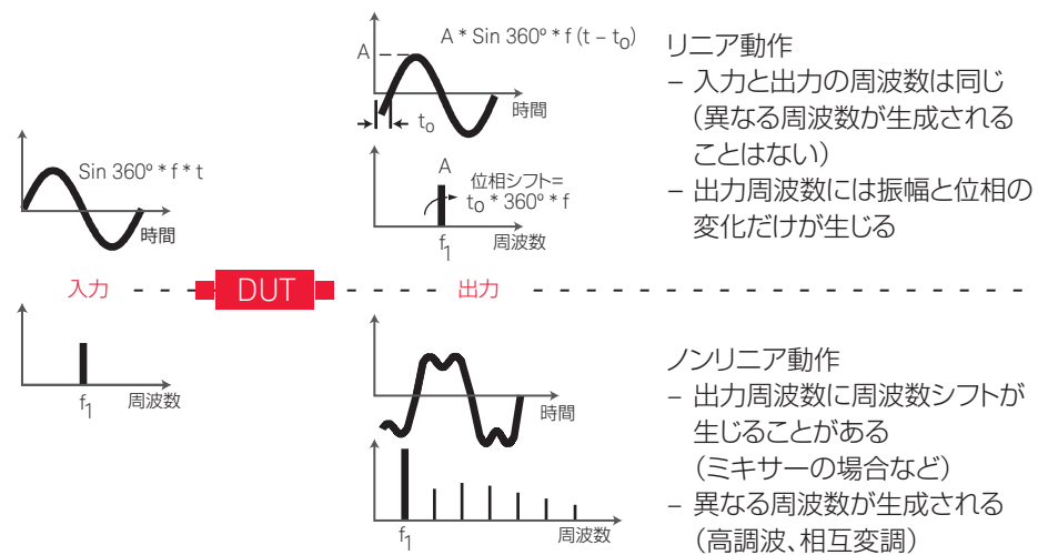
図1. リニア動作とノンリニア動作
