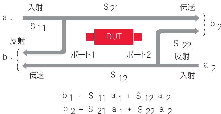
図16. H、Y、Zパラメーターの限界(Sパラメーターを使用する理由)
