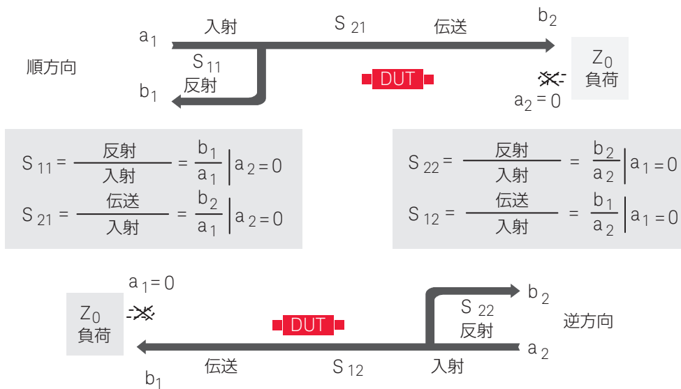
図17. Sパラメーターの測定
