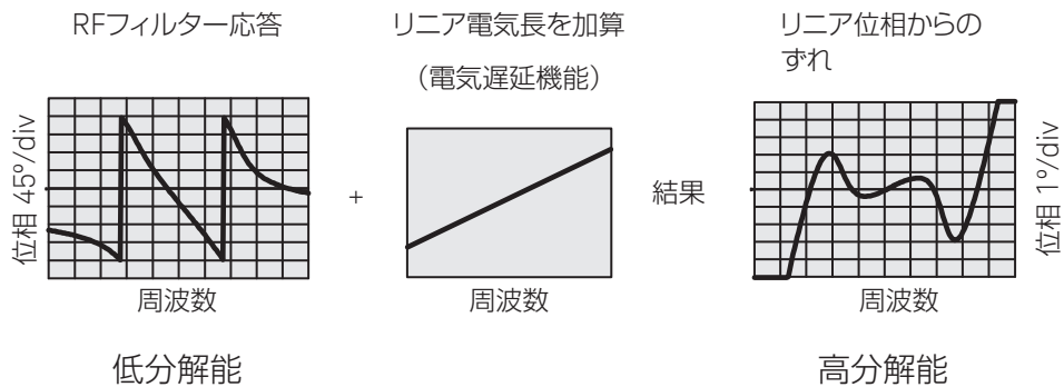
図13. リニア位相からのずれ
