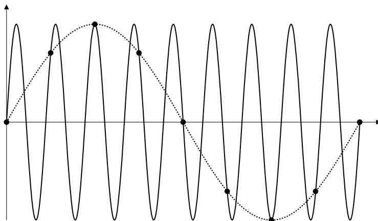
Abbildung 35 Aliasing
