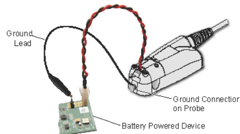
Abbildung 47 Messungen an batteriebetriebenen Geräten mit Tastkopf N2820A
