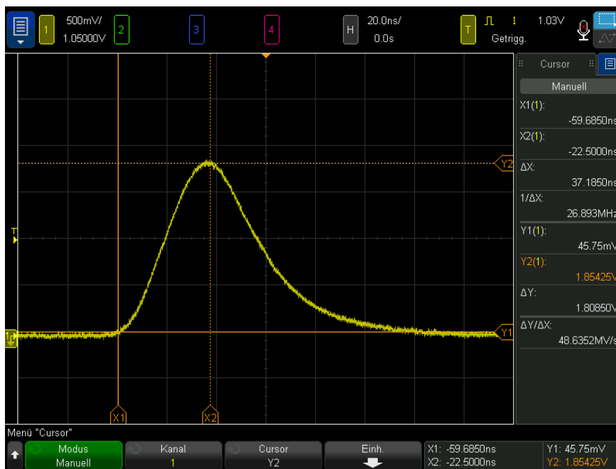
Abbildung 42 Zur Messung von anderen Impulsbreiten als mittleren Schwellenwertpunkten verwendete Cursor
