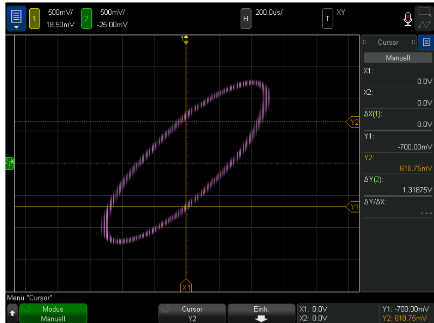
Abbildung 4 Phasendifferenzmessungen, automatisch und mit Cursors
