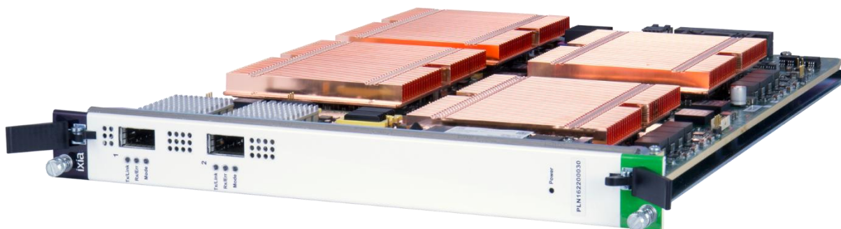
CloudStorm 2 x 100GE (CS100GE2Q28NG) load module
