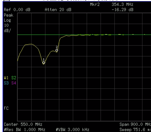
图 24 测量滤波器的回波损耗
