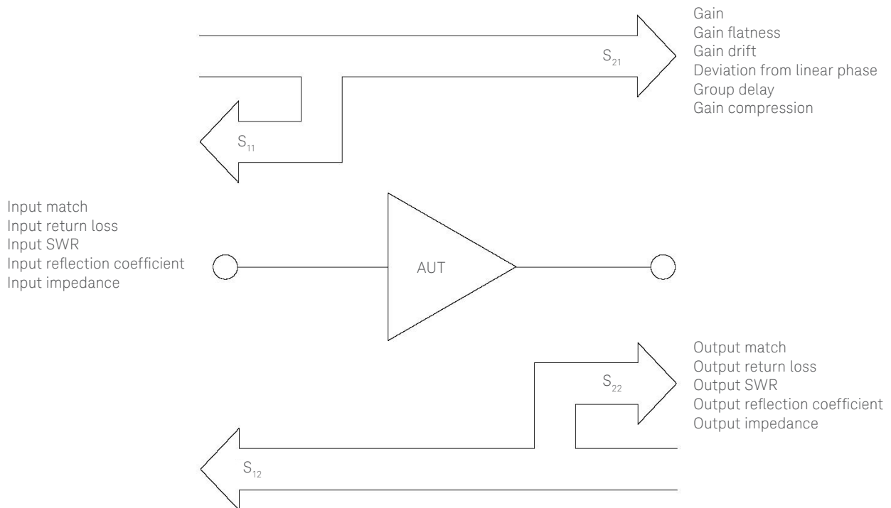
Figure 1. Amplifier parameters
